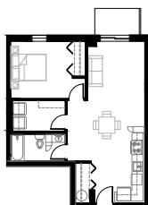
Logement type F - 1cc 65 m 2
