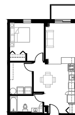
Logement type P - 1cc 65 m 2
