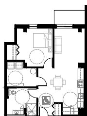
Logement type E - 1cc 75 m 2 - Adapté
