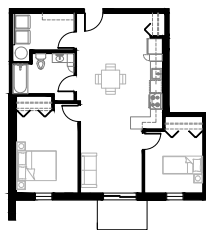
Logement type A - 2cc 82 m 2
